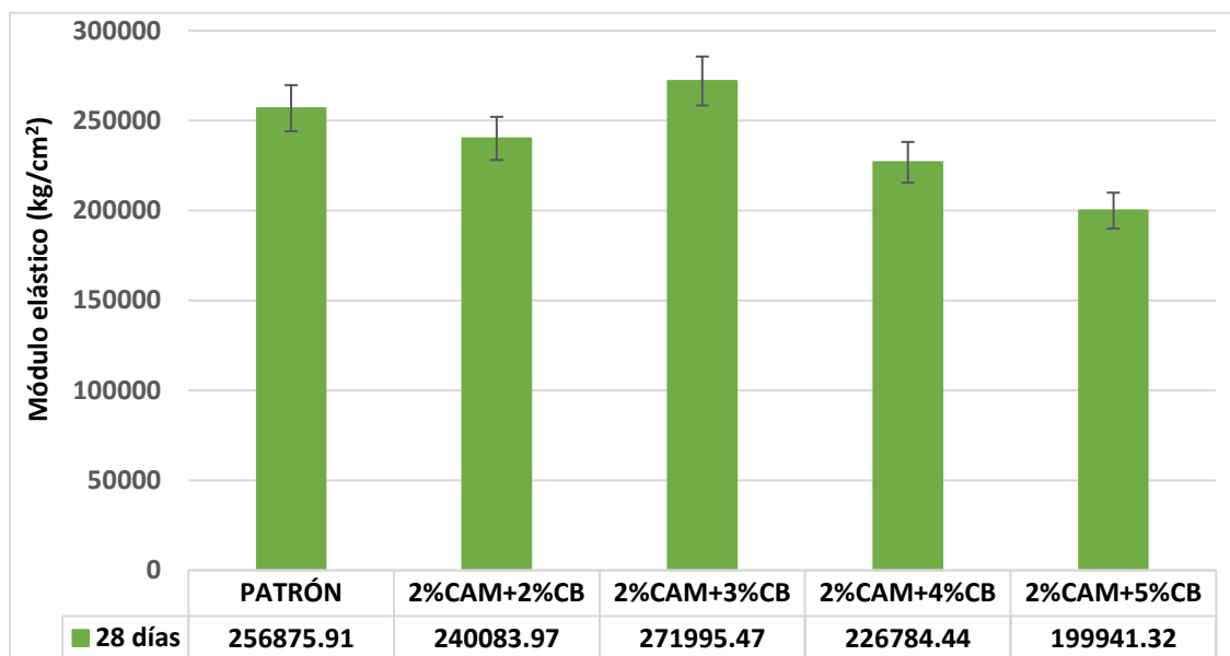
Fig. 21 Resultados de módulo de elasticidad de concreto de f'c=210 kg/cm 2 con incorporación de Ceniza de aserrín y bambú
