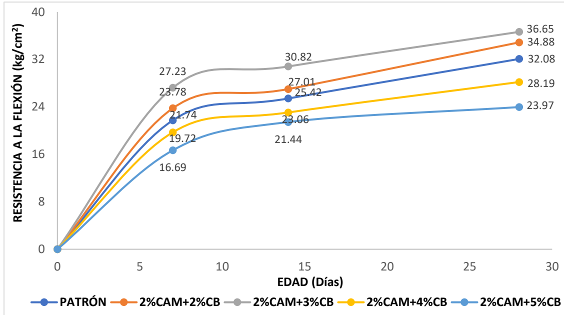
Fig. 17 Resultados de ensayo de resistencia a la flexión de concreto de f'c=210 kg/cm 2 con incorporación de Ceniza de aserrín y bambú
