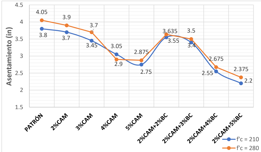
Fig. 3 Resultados de ensayo de slump
