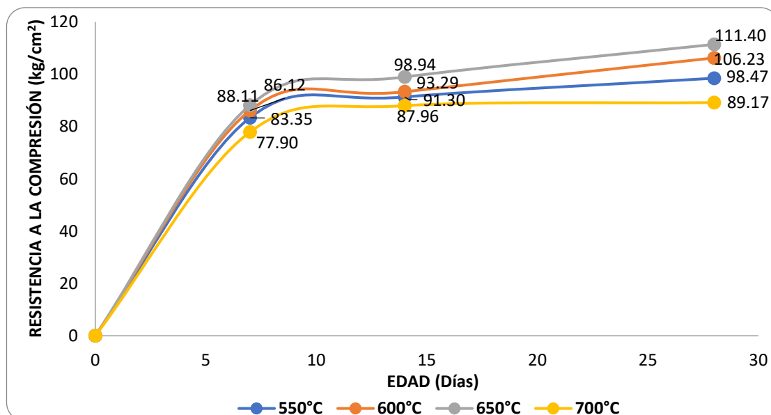
Fig. 6 Resultados de ensayo de compresión simple para la obtención de temperatura óptima de quemado de ceniza de bambú
