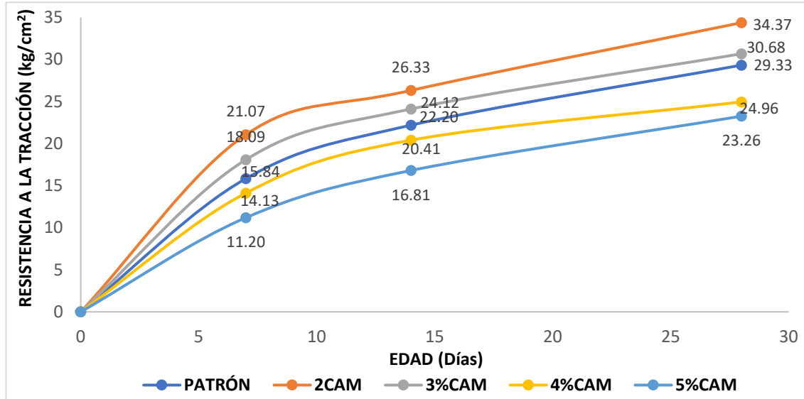
Fig. 11 Resultados de ensayo de resistencia a la tracción de concreto de f'c=210 \text{ kg/cm}^2 con sustituto de Ceniza de aserrín de madera
