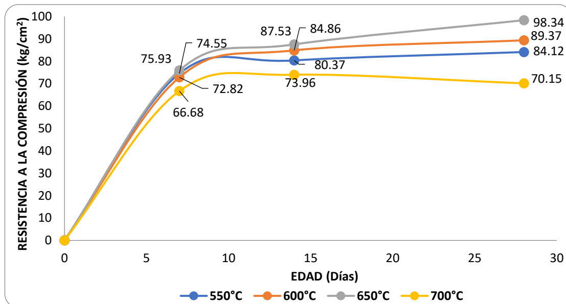
Fig. 5 Resultados de ensayo de compresión simple para la obtención de temperatura óptima de quemado de Ceniza de Aserrín de madera
