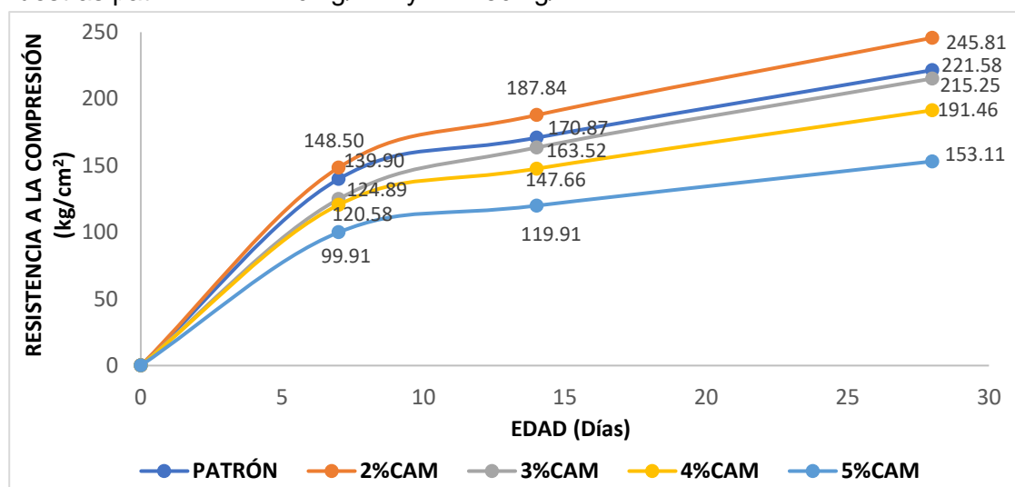
Fig. 7 Resultados de ensayo de resistencia a la compresión de concreto de f'c=210 kg/cm 2 con sustituto de Ceniza de aserrín de madera
