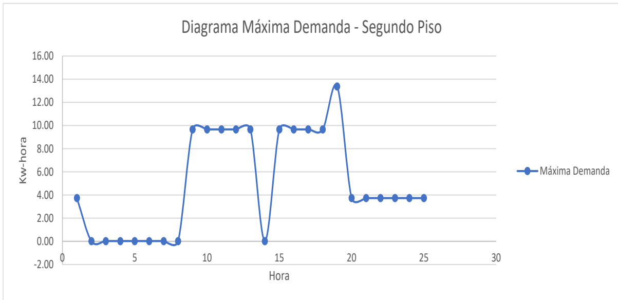
Figura. 15. Diagrama de carga diaria segundo piso – edificio de ingeniería.
