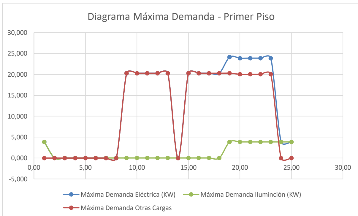
Figura. 12. Diagrama de carga diaria iluminación, otras cargas primer piso – edificio de ingeniería.
