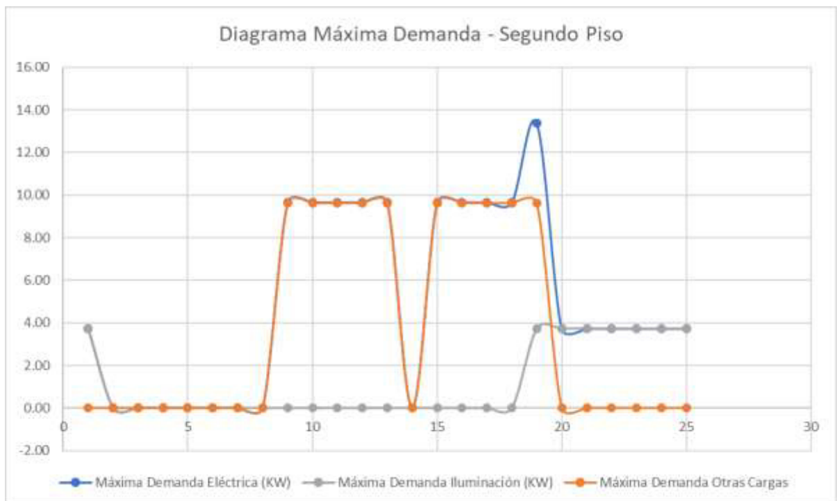
Figura. 14. Diagrama de carga diaria iluminación, tras cargas segundo piso – edificio de ingeniería.
