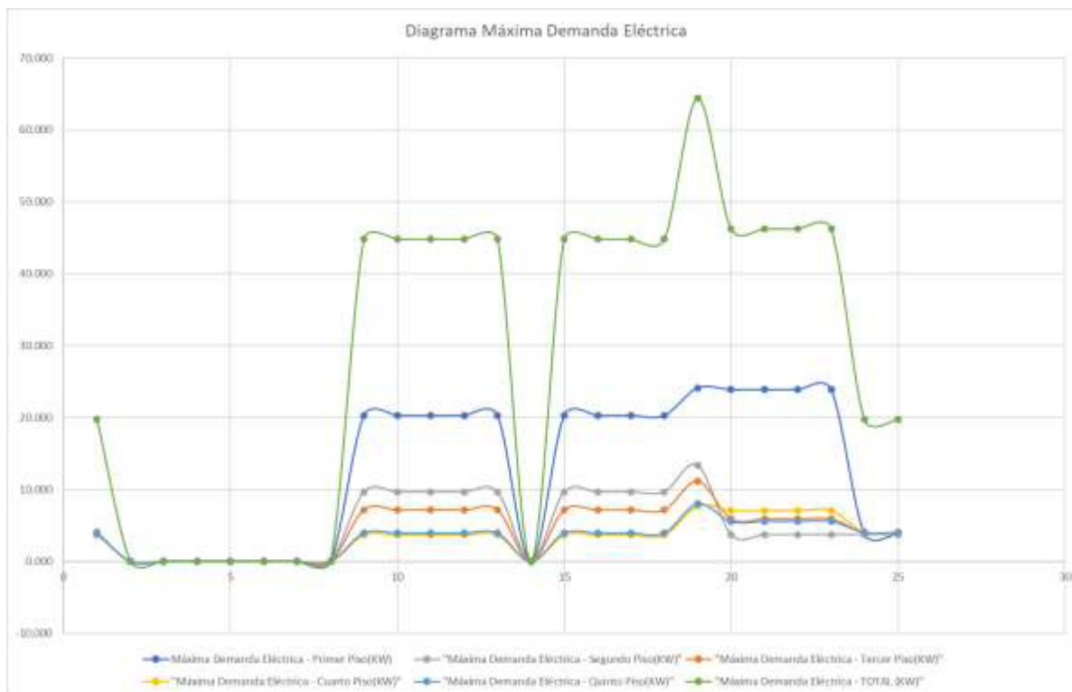
Figura. 22. Diagrama de carga diaria total – edificio de ingeniería
