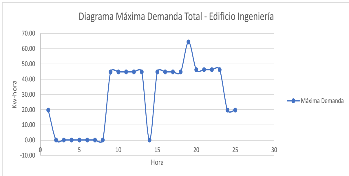
Figura. 23. Diagrama de carga diaria total – edificio de ingeniería.
