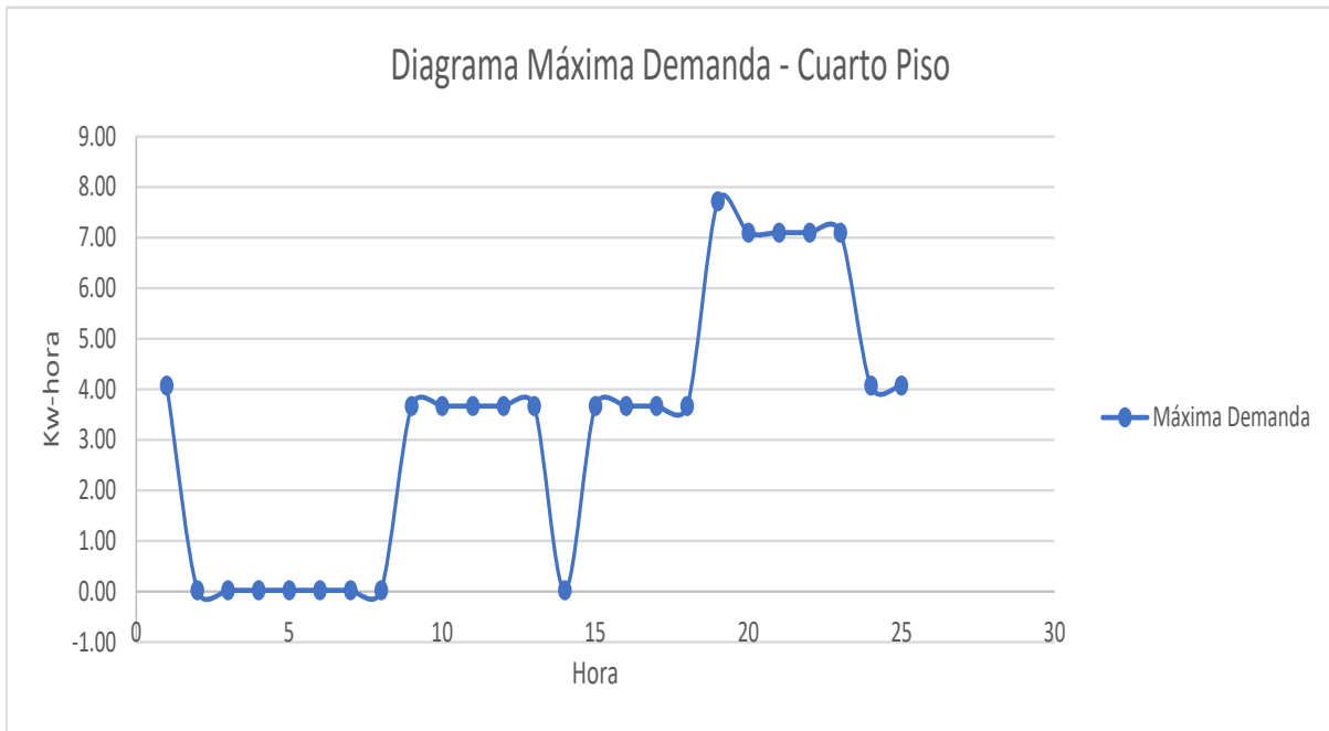
Figura. 19 Diagrama de carga diaria cuarto piso – edificio de ingeniería
