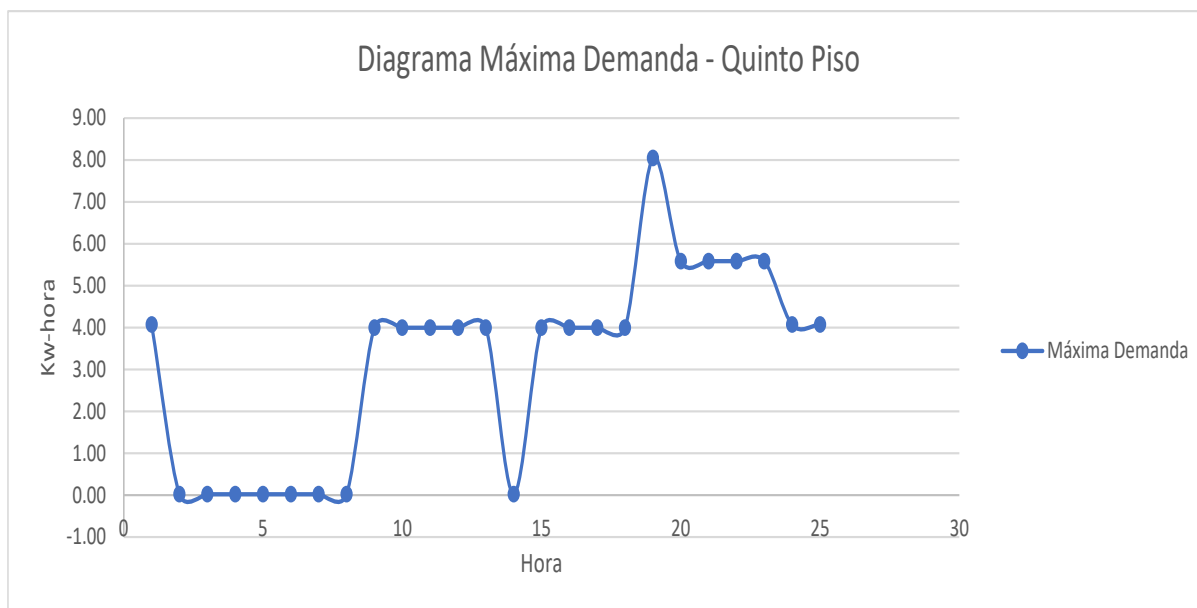
Figura. 21. Diagrama de carga diaria quinto piso – edificio de ingeniería.
