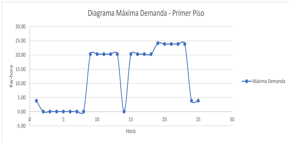
Figura. 13. Diagrama de carga diaria primer piso – edificio de ingeniería.
