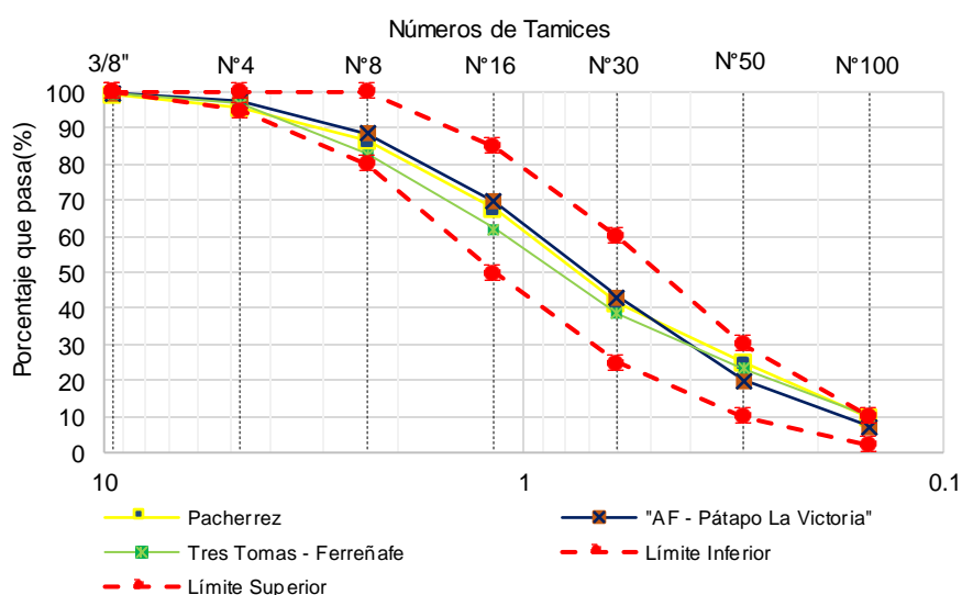
Fig. 1. Granulometría para el agregado fino extraído de diversas canteras.
