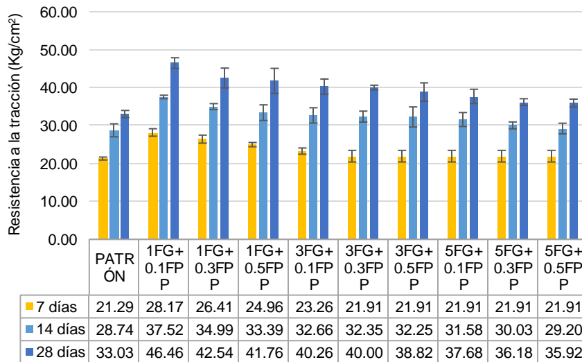
Fig. 9. Resistencia a la tracción del mortero con la combinación de FG + FPP en dosificación 1:3.
