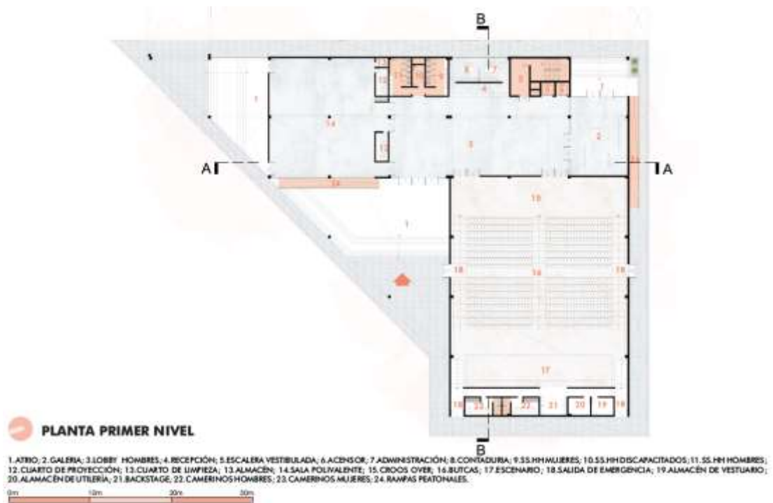
Figura 63: Planta primer nivel bloque auditorio Elaboración: Propia
