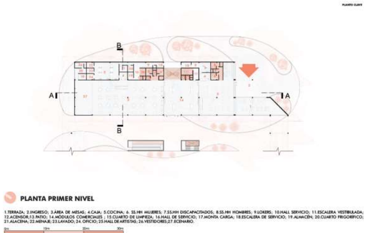
Figura 68: Planta primer nivel bloque de servicios complementarios Elaboración: Propia
