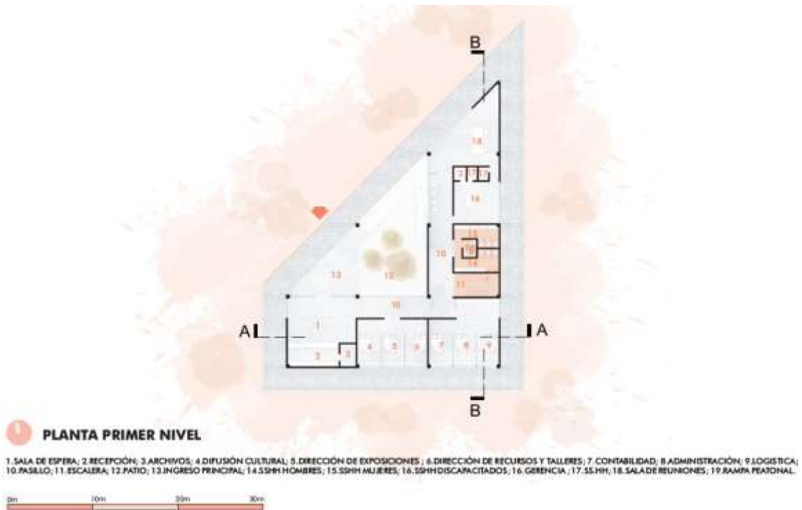
Figura 72: Planta primer nivel bloque administrativo
