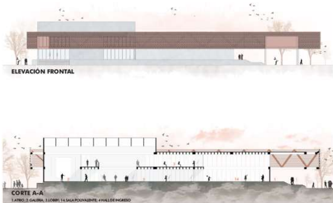
Figura 65: Corte y elevación bloque auditorio Elaboración: Propia
