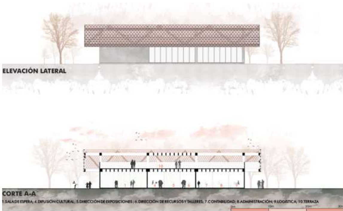
Figura 72: corte y elevación de bloque administrativo Elaboración: Propia
