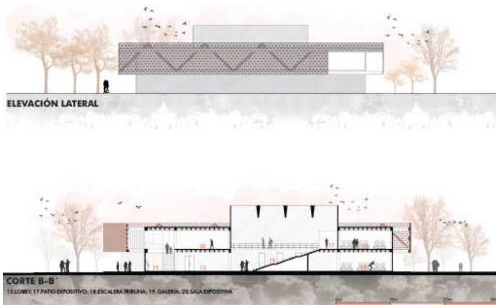
Figura 62: corte y elevación bloque Museo Elaboración: Propia
