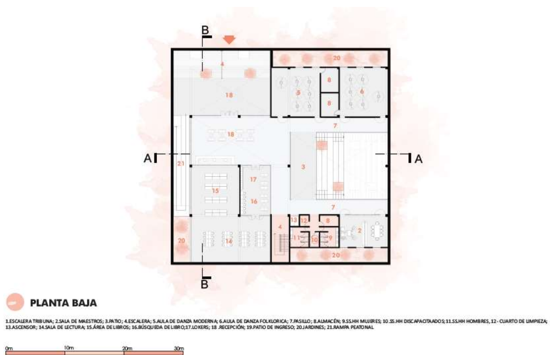
Figura 54: Planta baja bloque de talleres
