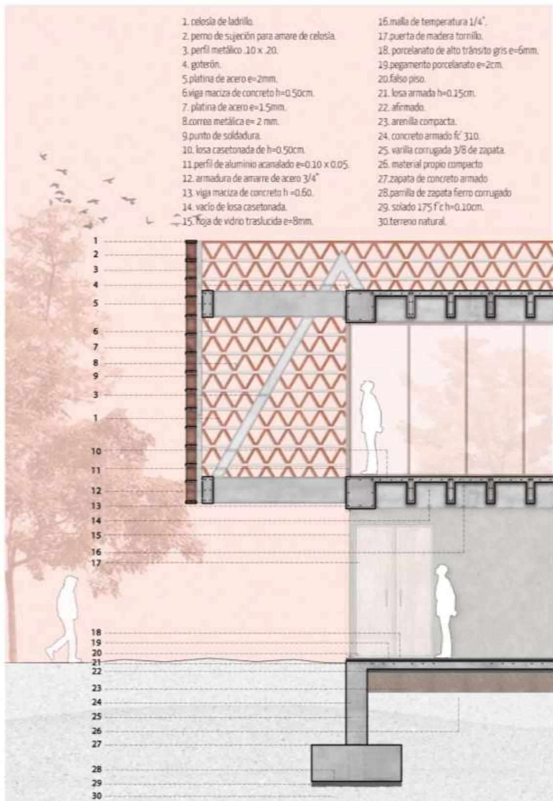
Figura 74: corte constructivo Elaboración: Propia
