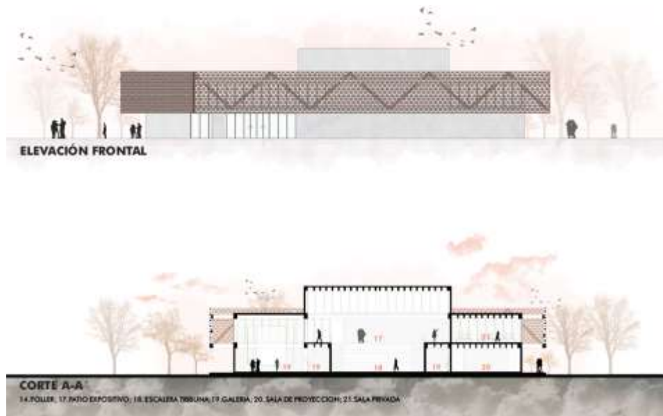
Figura 61: corte y elevación bloque Museo Elaboración: Propia
