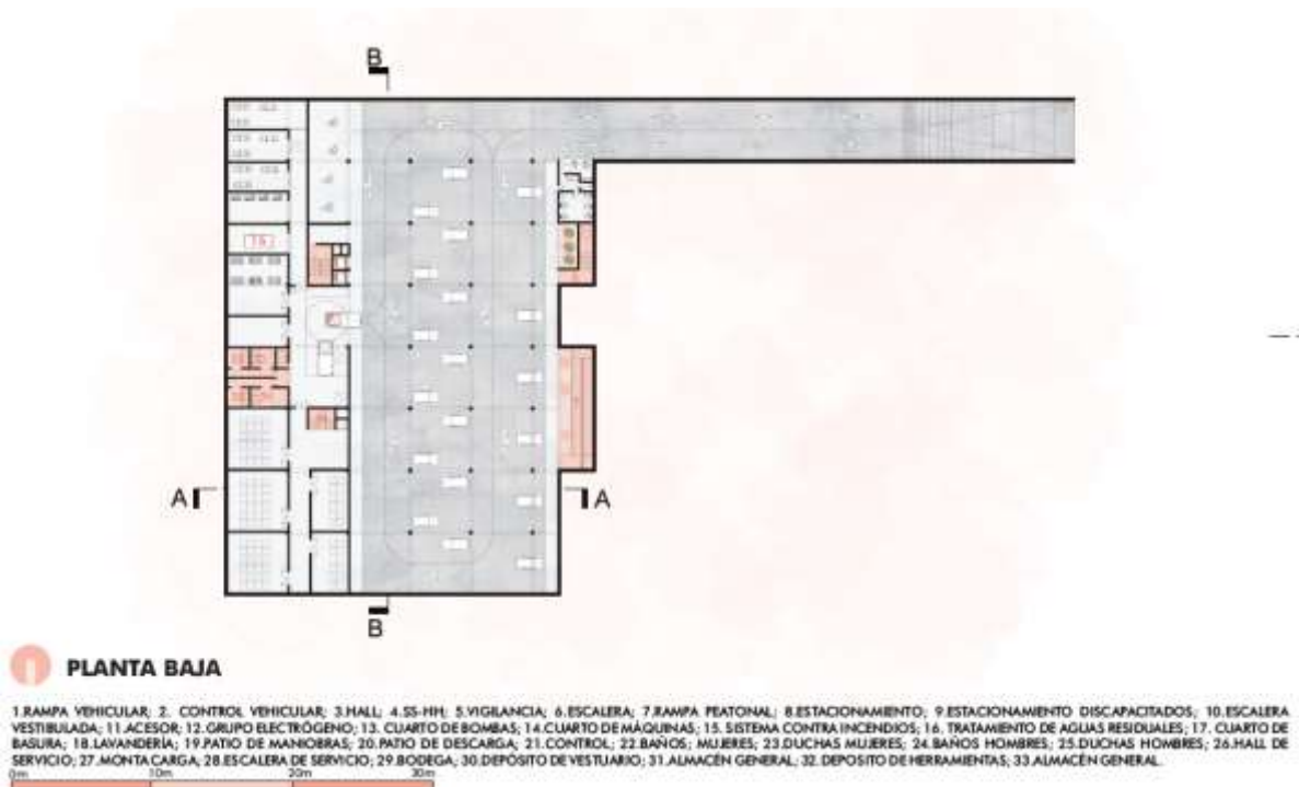
Figura 67: Planta baja estacionamiento bloque de servicios complementarios Elaboración: Propia
