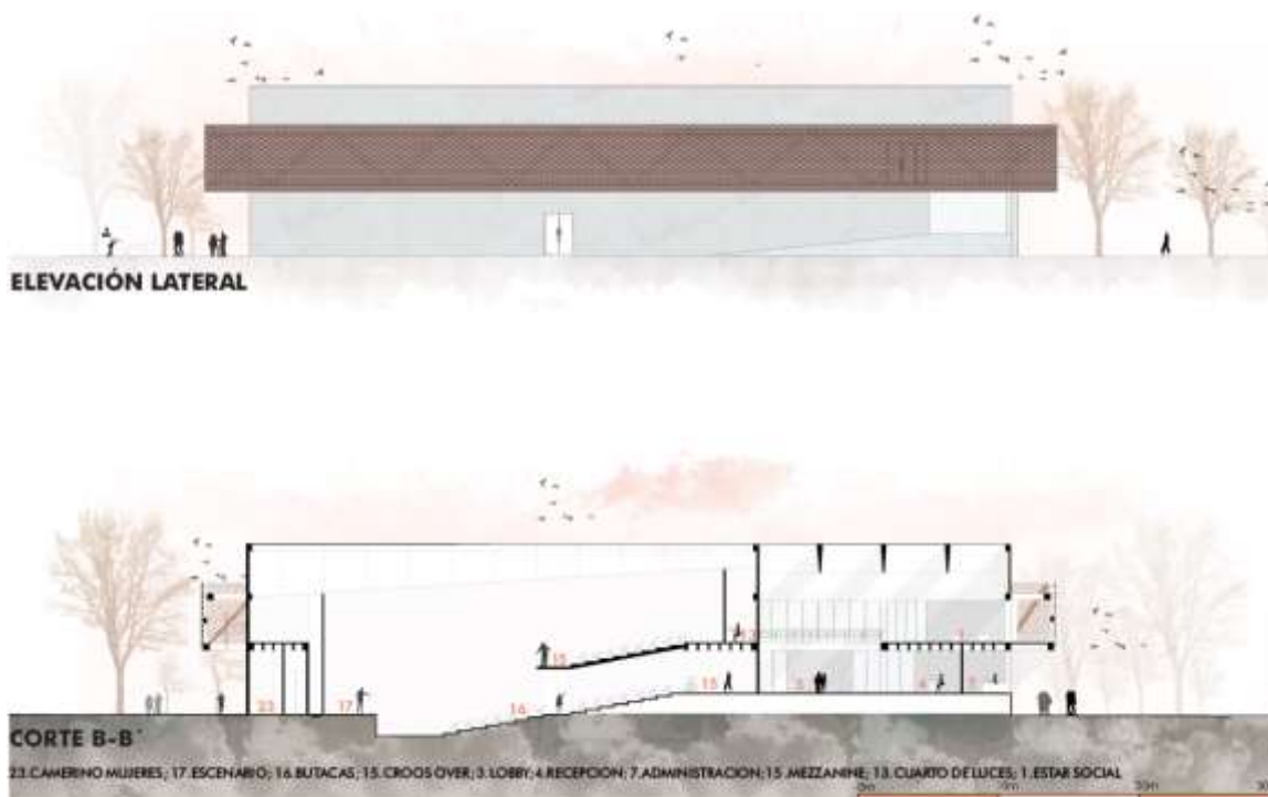
Figura 66: Corte y elevación bloque auditorio Elaboración: Propia
