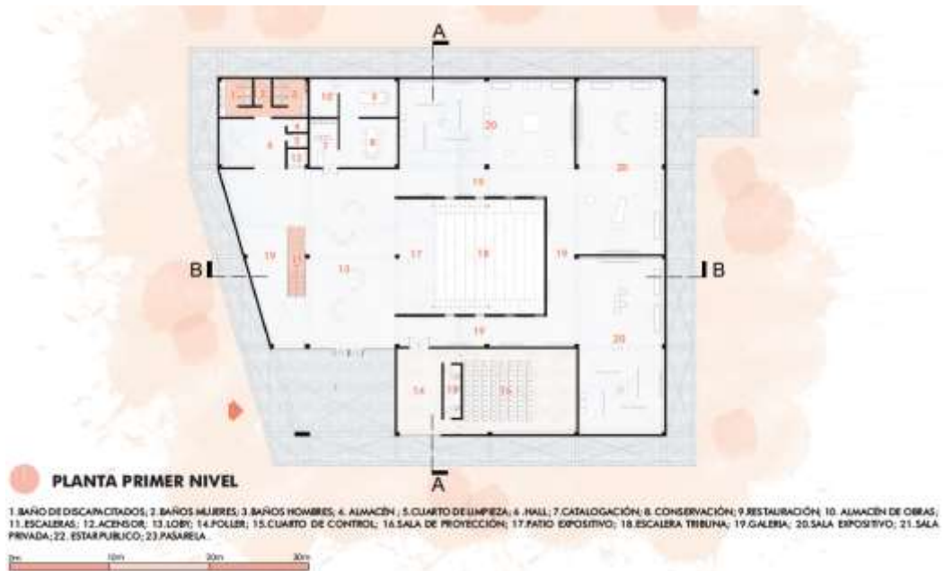
Figura 59: Planta primer nivel bloque Museo Elaboración: Propia
