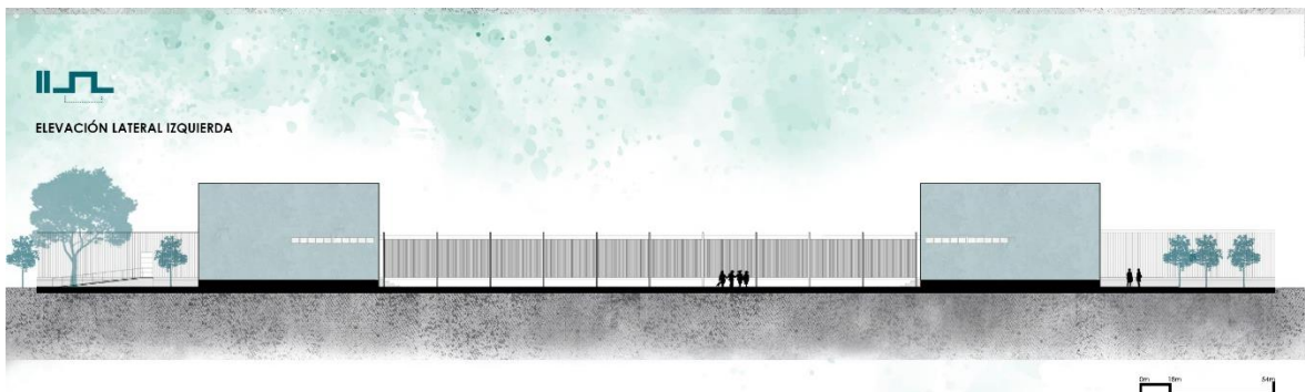
Figura 53 Elevación lateral izquierda Elaboración Propia
