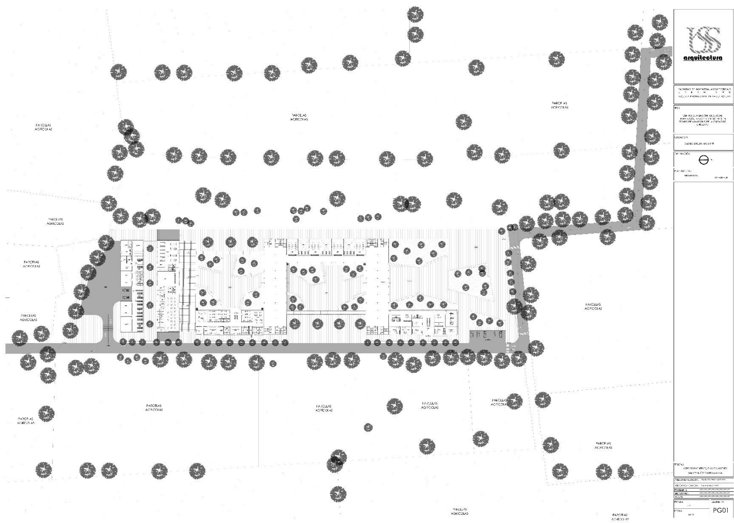
Figura 47 Planta Arquitectónica Primer Nivel Elaboración Propia
