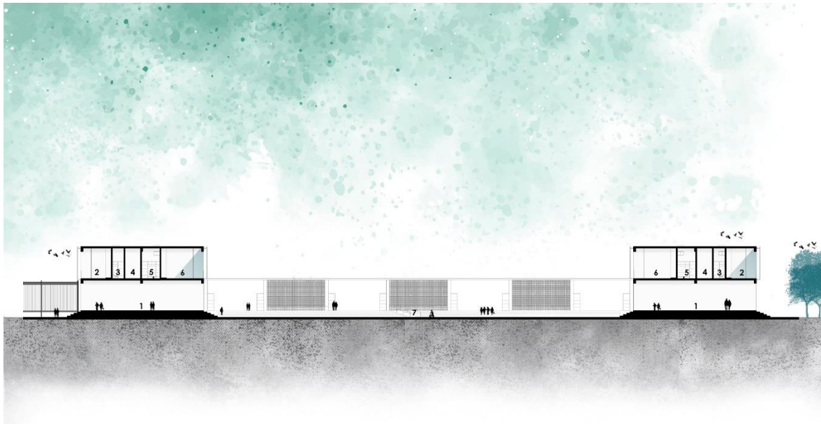
CORTE C - C' +1.00 | +4.20 | +9.40 1. Acceso principal; 2. Dormitorio 3. Ss.hh; 4. Pasillo; 5. Ss.hh; 6. Dormitorio; 7. Plaza de integración.
