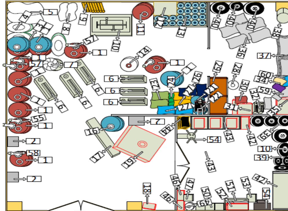
Figura 17: Diseño o layout del área de combustibles antes
