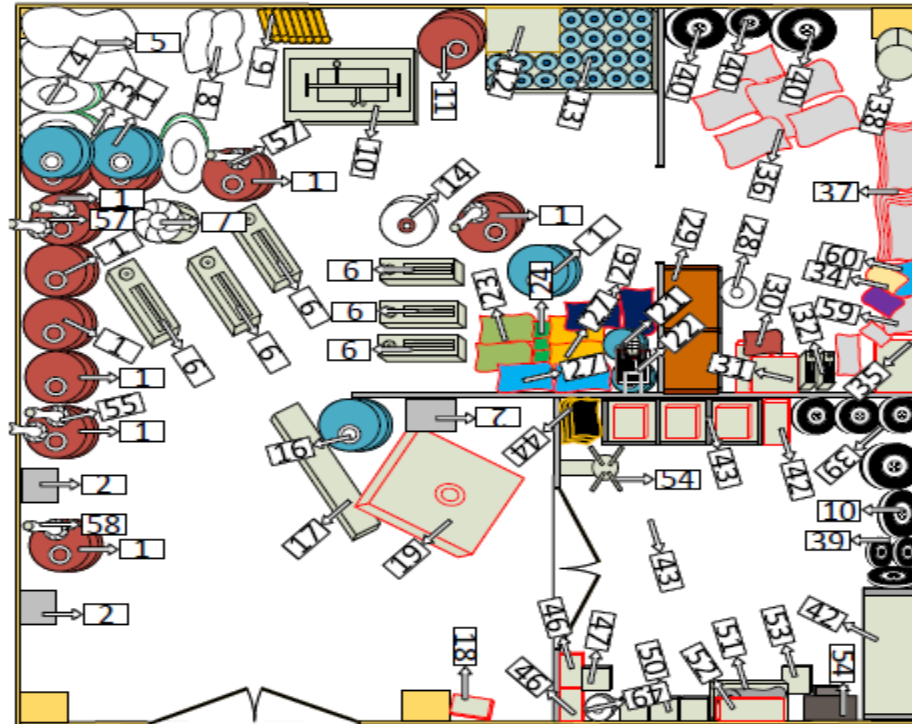
Figura 25: Diseño o layout del área de combustible
