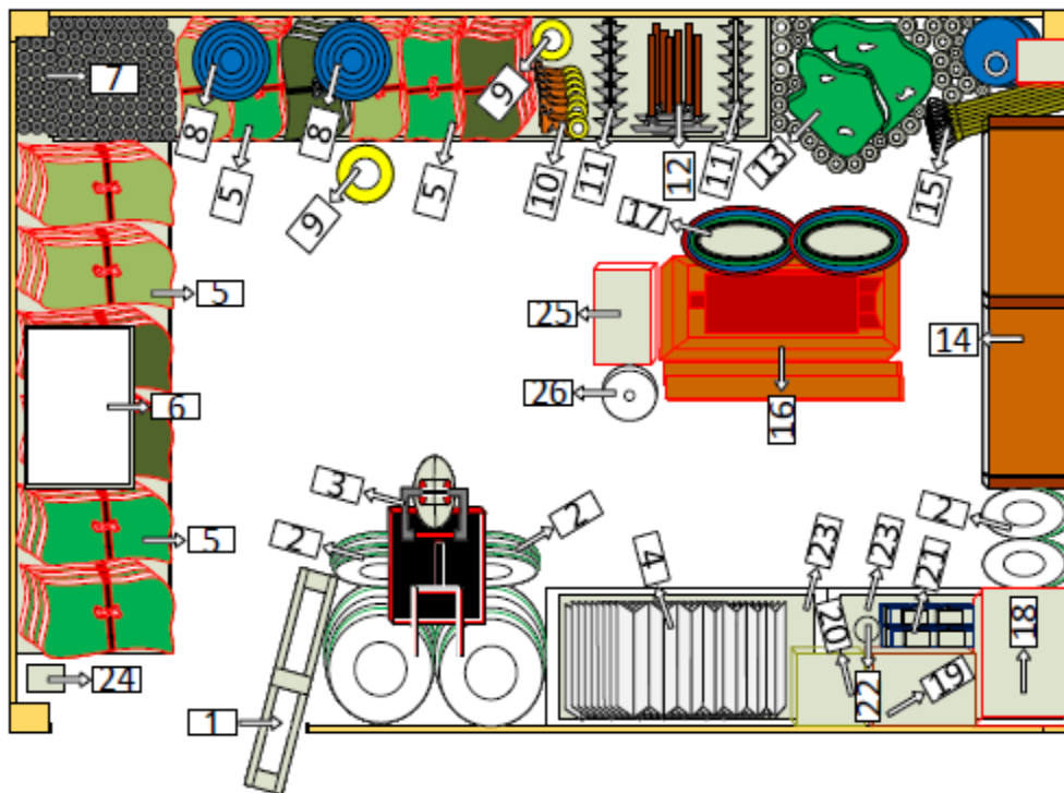
Figura 27: Diseño o layout del área de zona a - agroquímicos
