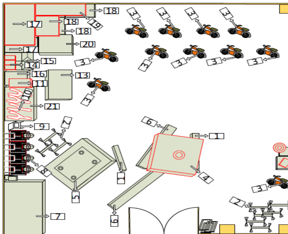
Figura 15: Diseño o layout del área de patrimonio antes
