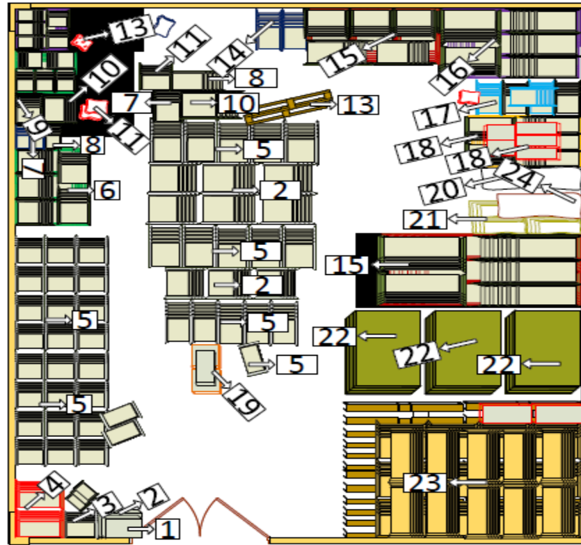
Figura 14: Diseño o layout del almacén 3 antes
