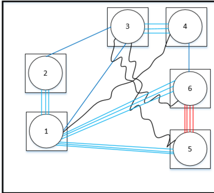
Figura 436: Diagrama de Hilos Mejorado.
