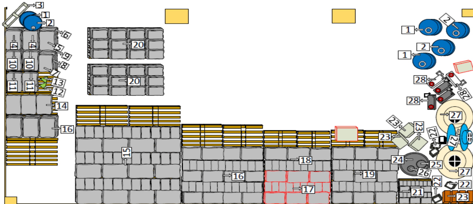
Figura 16: Diseño o layout del área de patio antes
