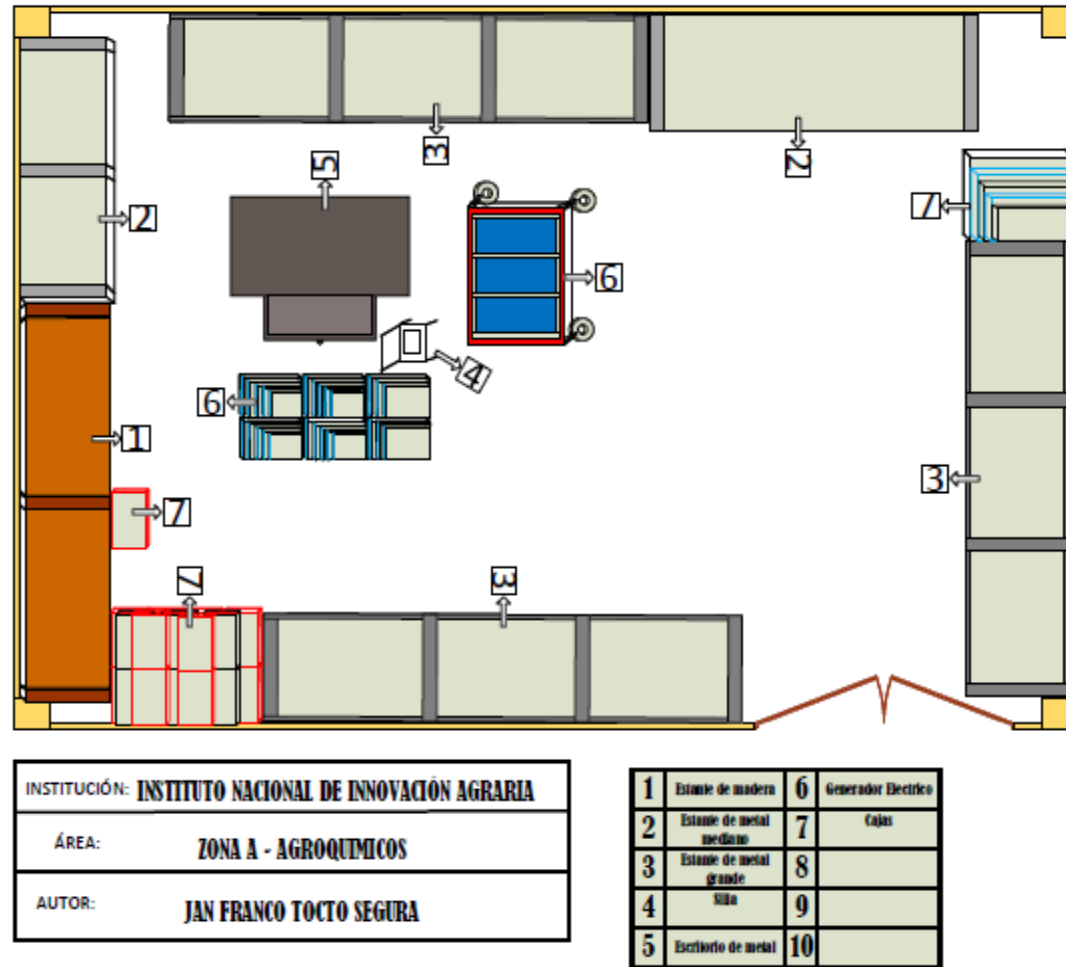
Figura 18: Diseño o layout del área de zona a - agroquímicos antes
