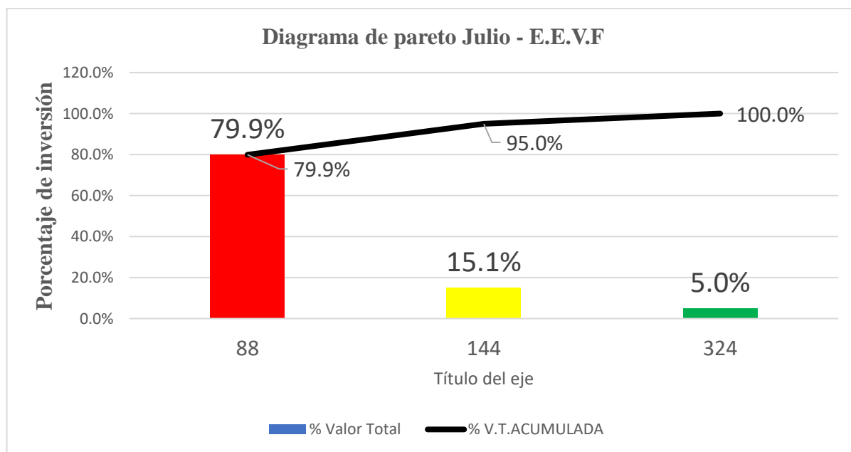
Gráfico 27: Diagrama de pareto Julio– E.E.V.F
