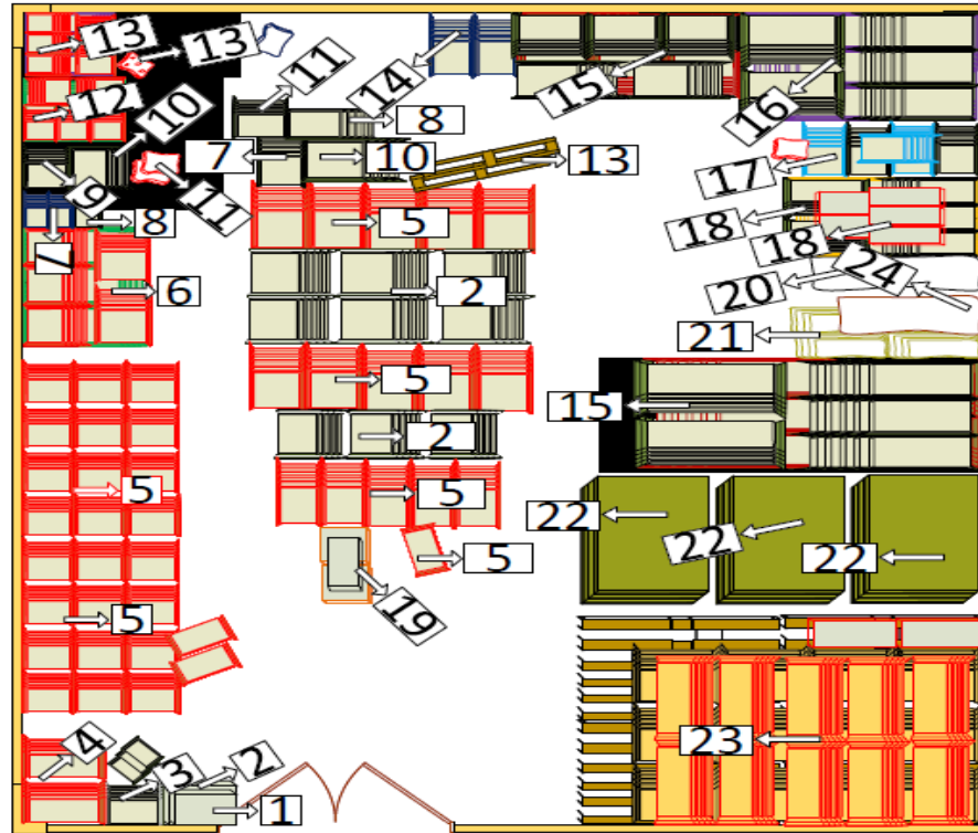
Figura 22: Diseño o layout del área de almacén 3
