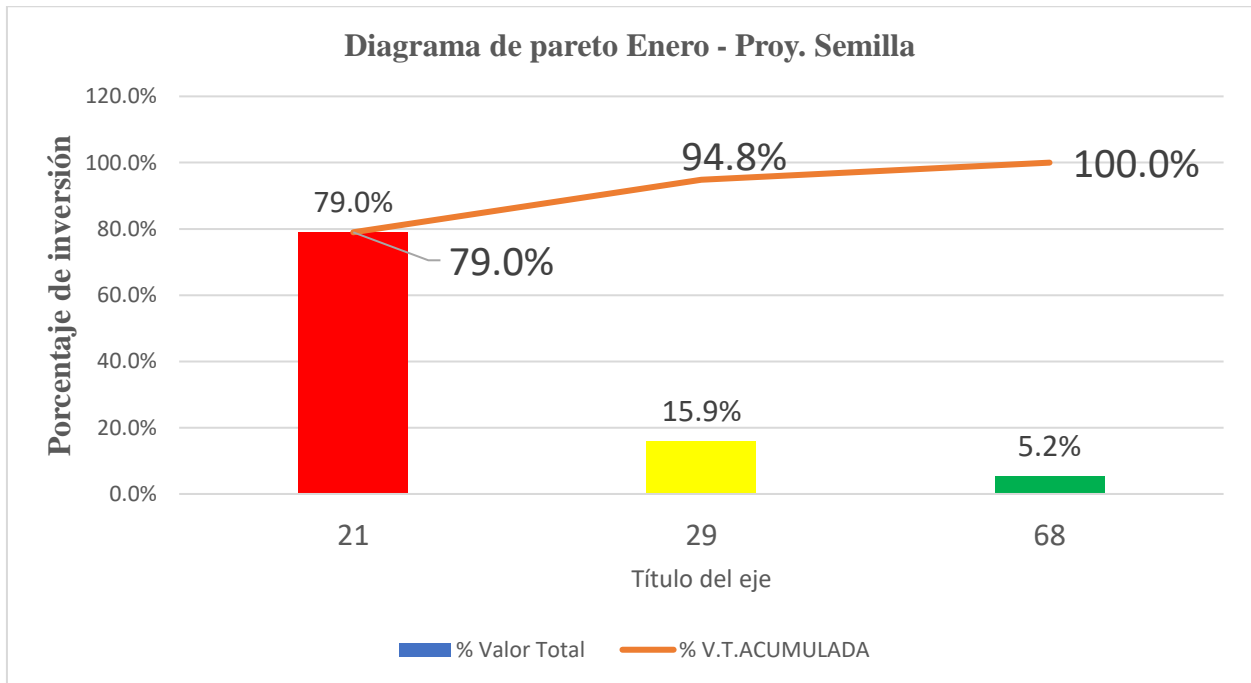
Gráfico 12: Diagrama de pareto Enero – Proyecto Semilla
