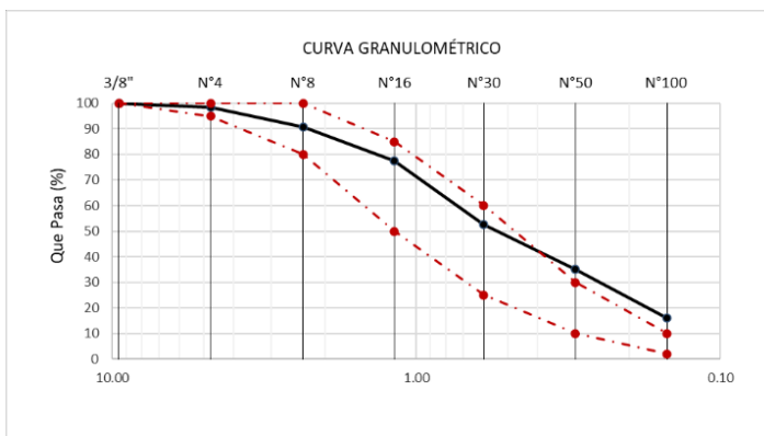
Fig. 3. Curva granulométrica AF
