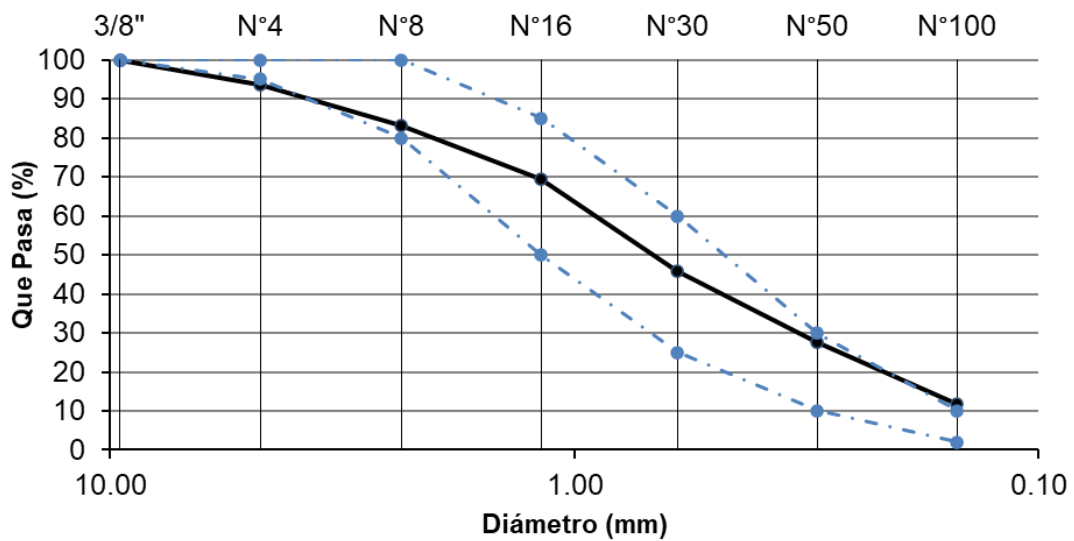
Fig. 4. Curva granulométrica del agregado fino Cantera Pacherres – Pucalá.
