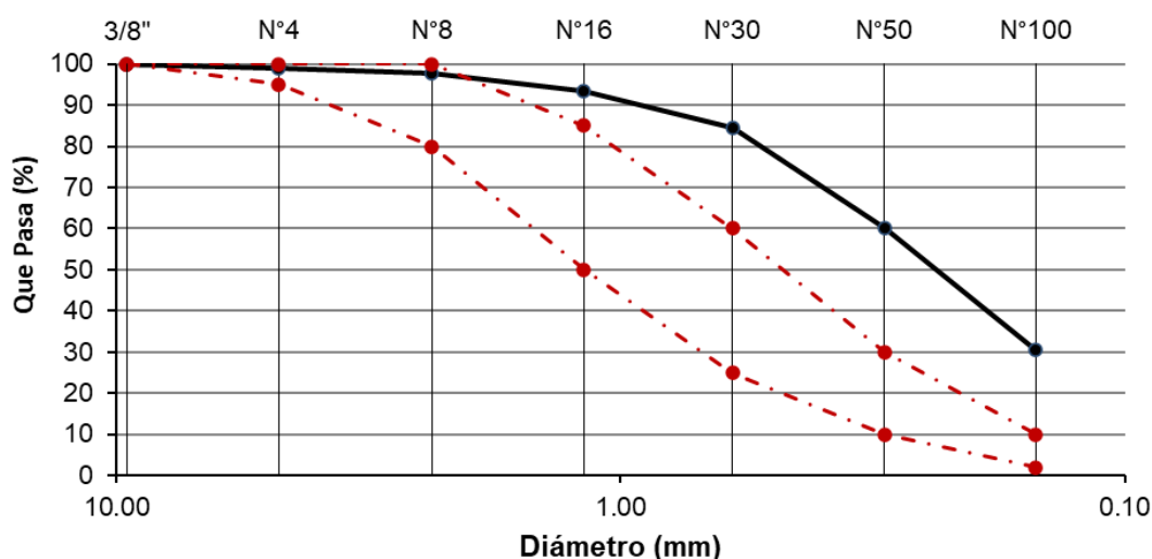
Fig. 12. Curva granulométrica de la ceniza de bagazo saccharum officinarum .
