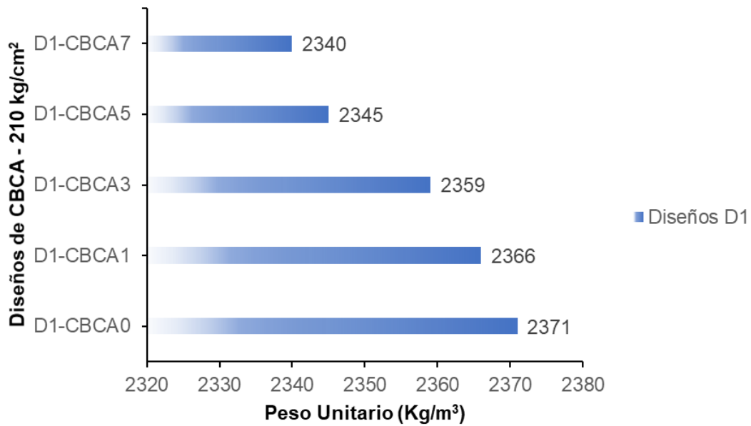
Fig. 17. Resultados del peso unitario para las mezclas concreto f'c : 210 kg/cm 2 (D1).
