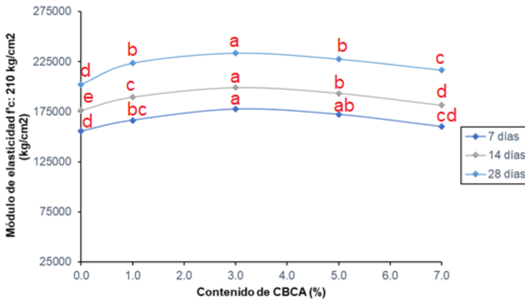
Fig. 27. Resultados de módulo de elasticidad para los concretos de f'c 210 kg/cm^2 (D1).
